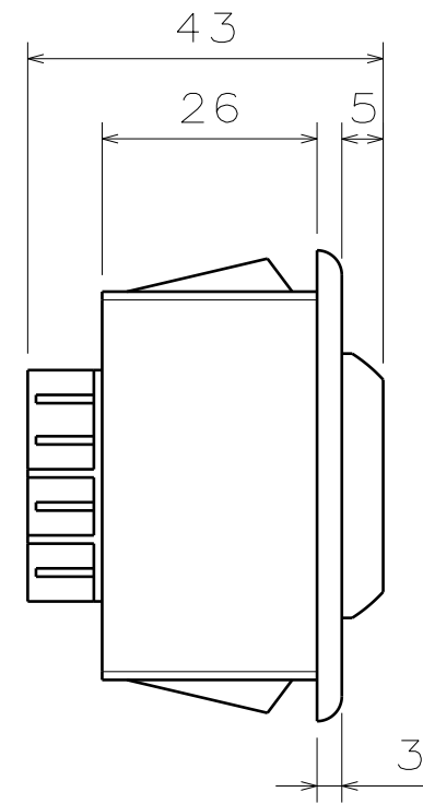
Left view Scale: 1:1
